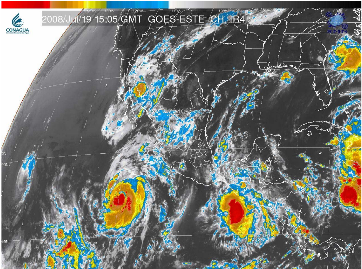
Imagen en canal Infrarrojo del satélite GOES-E del 19 de julio a las 1505 GMT Huracán "Fausto" al Sur de la Península de Baja California
