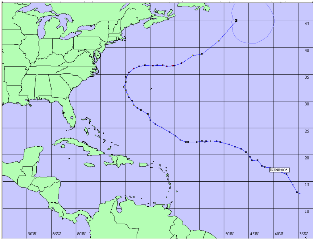
Trayectoria del Huracán "Irene" Del 4 al 18 de agosto de 2005
